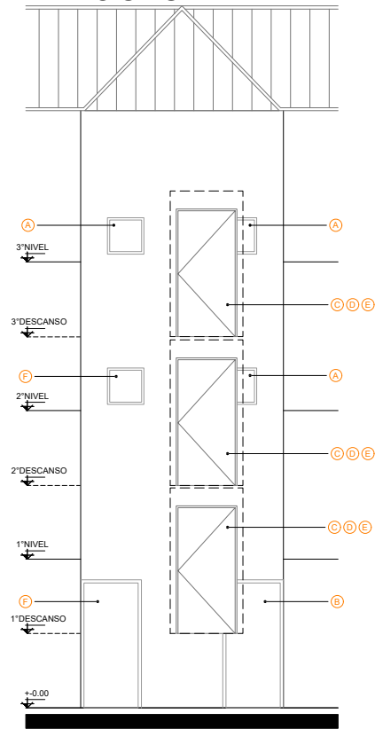
FACHADA EXISTENTE
