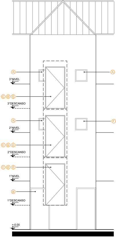
FACHADA EXISTENTE
