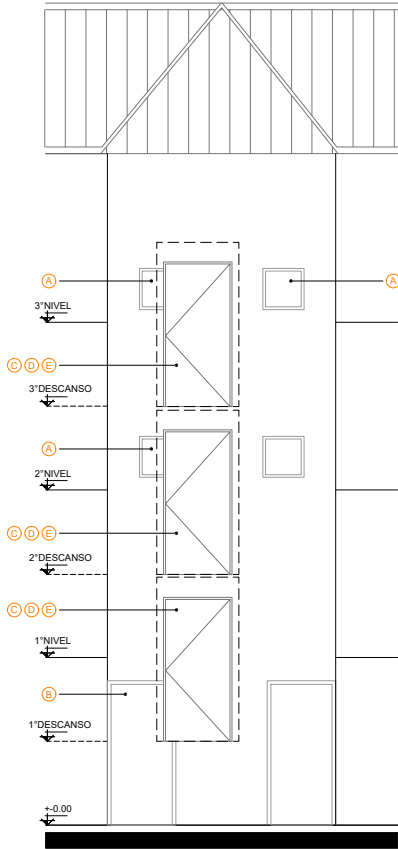
FACHADA EXISTENTE
