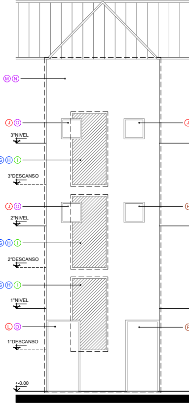
FACHADA PROYECTO
