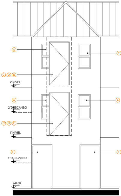
FACHADA EXISTENTE
