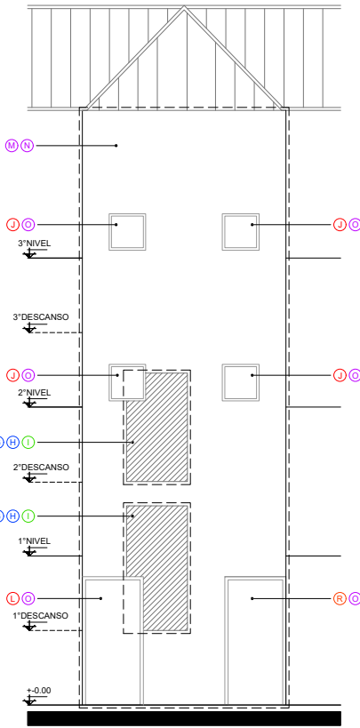
FACHADA PROYECTO
