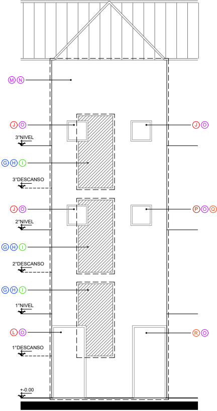
FACHADA PROYECTO
