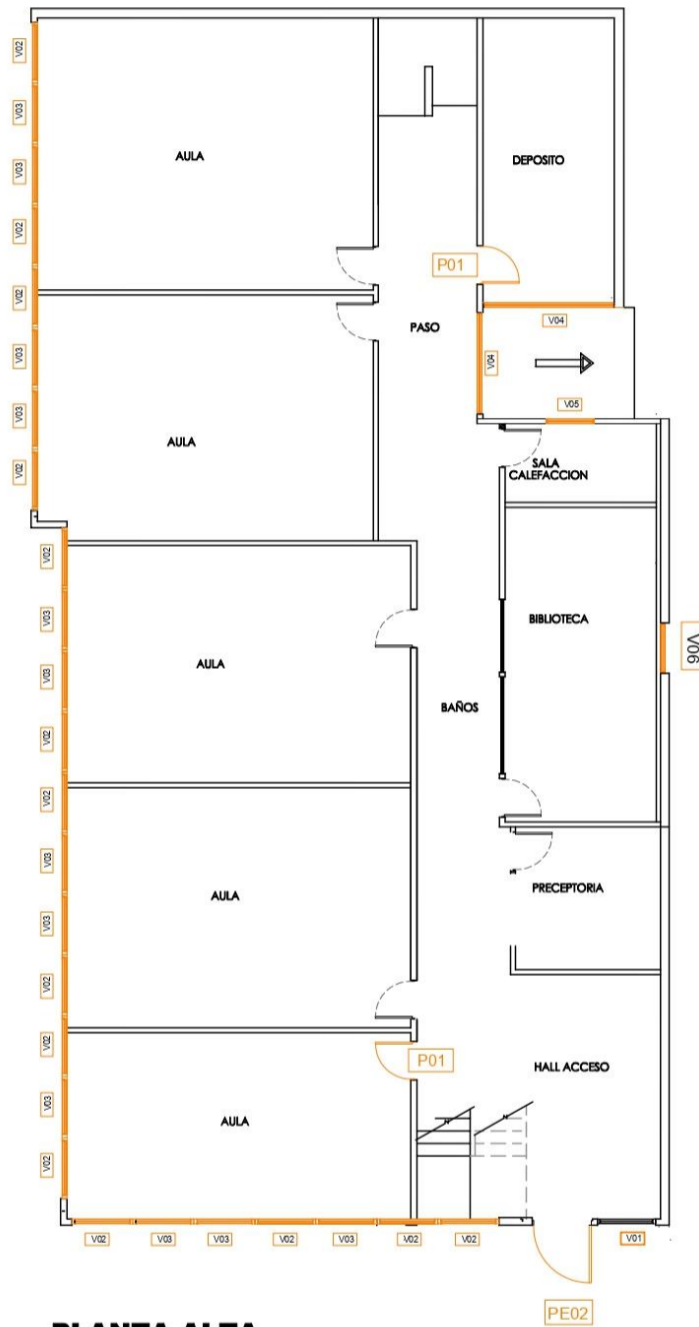
PLANTA ALTA
